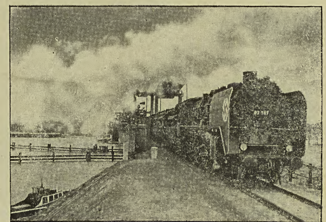
Rügen ist keine Insel mehr! — In Anwesenheit des schwedischen und norwegischen Gesandten in Berlin und vieler führender Persönlichkeiten der nordischen Staaten sowie zahlreicher Vertreter von Partei und Staat, fand die Eröffnung des Eisenbahnverkehrs über den Rügendamms statt. Die Eröffnung des Fahrdamms wird erst in einigen Monaten erfolgen.
