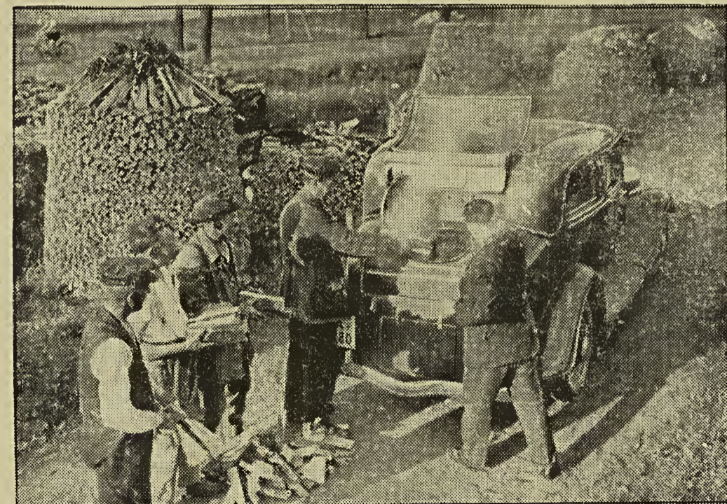
Mit Holzgas über die Alpen. — Ein 3,3 Liter Personenkraftwagen mit Holzgasantrieb, wie er zur Internationalen Alpenwertungsfahrt entsandt wurde. Bei der Prüfungsfahrt wurden innerhalb von acht Tagen zwölf Alpenpässe befahren, die Höhenunterschiede von 8 bis 1900 Meter aufwiesen. Das Fahrzeug blieb auf der ganzen Strecke störungsfrei.
