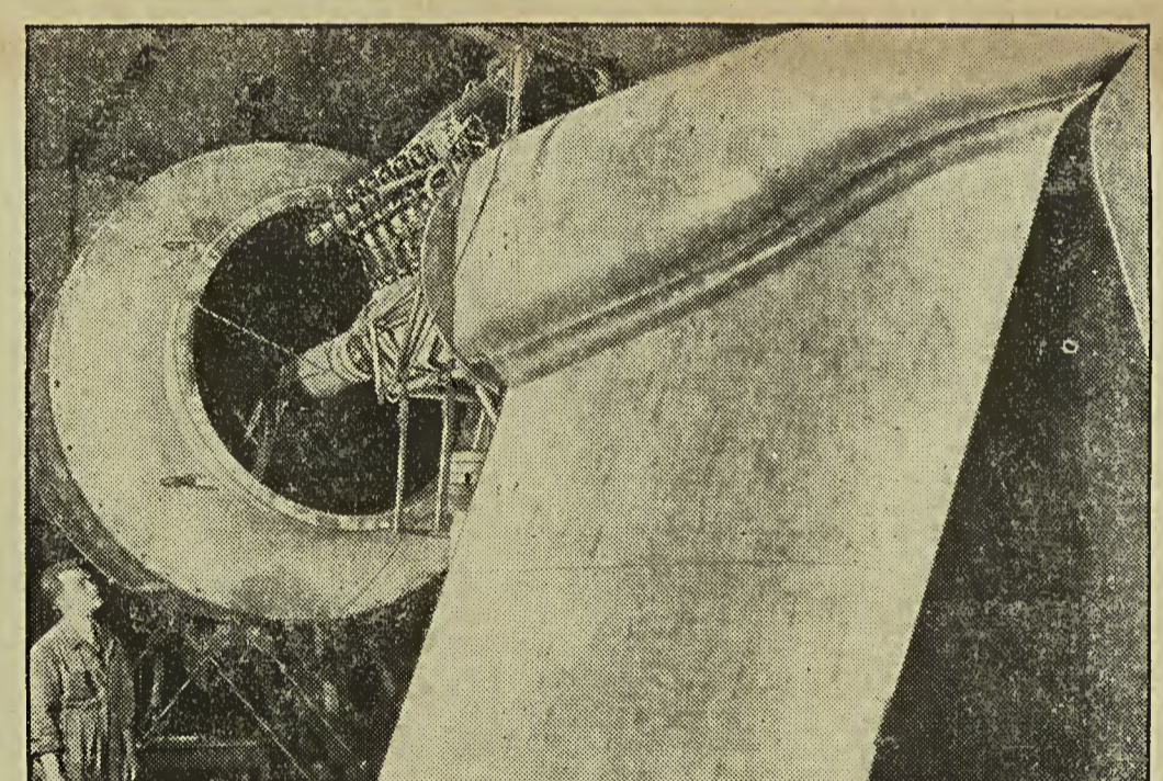
Im Motoren-Prüfstand. — In der deutschen Versuchsanstalt für Luftfahrt in Adlershof bei Berlin wird das gesamte Material, das in der deutschen Luftfahrtindustrie verwandt wird, einer genauesten Prüfung unterzogen.
