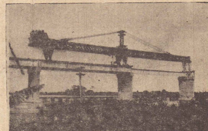
Em março deste ano (data da foto estampada acima) estavam prontos 135 metros de vigas de concreto pretendido e pré moldado. Note-se que em abril, ou seja no mês seguinte, 430 outros metros já haviam sido colocados (conforme foto do clichê com aqueles detalhes
