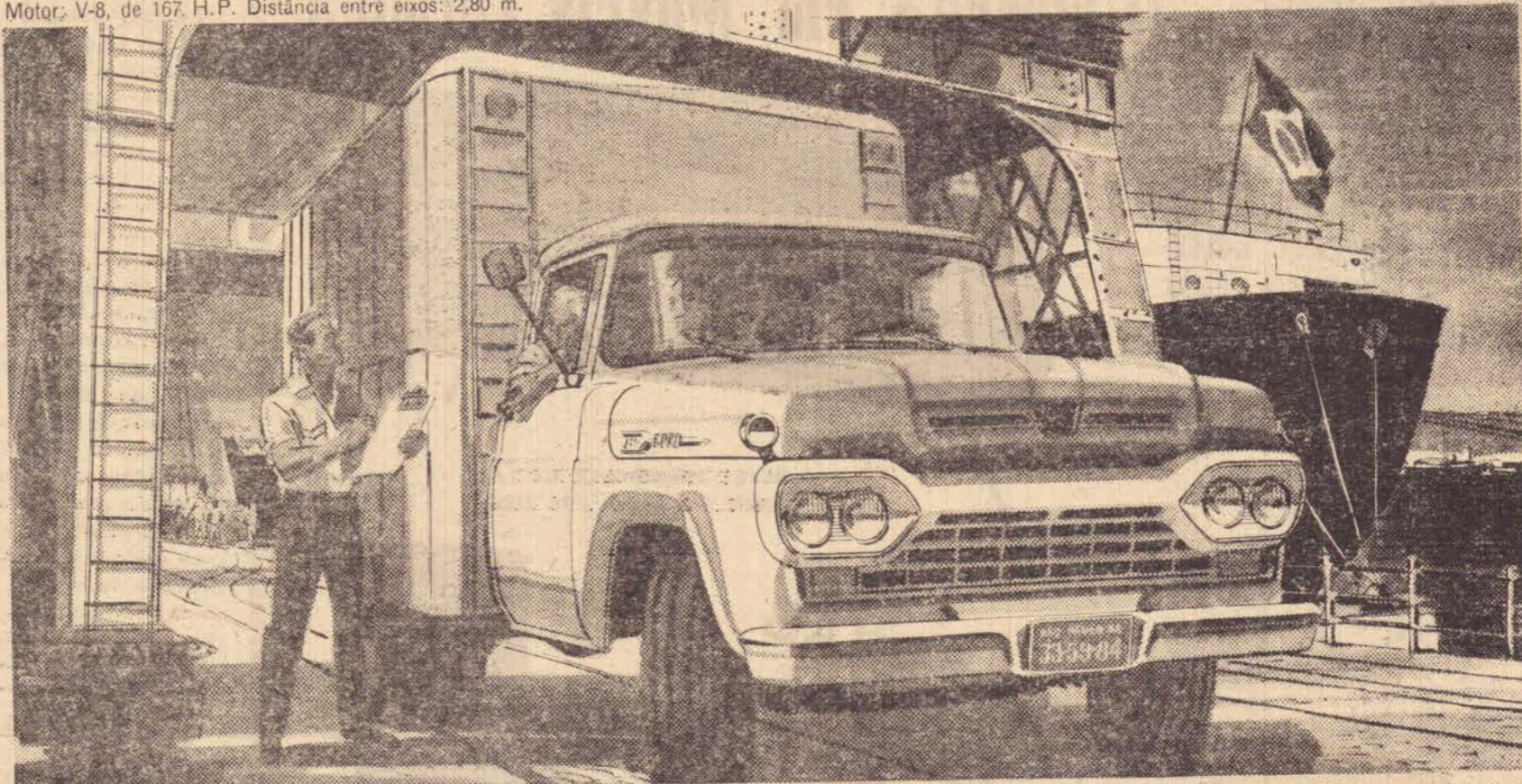
SUPER FORD F-350 — Único caminhão de tonelage média fabricado no Brasil, para o transporte de mercadorias relativamente leves, mas volumosas. Capacidade de carga: 2.670 kg Motor: V-8, de 167 H.P. Distância entre eixos: 3,30 m. Diferencial: reforçado, tipo hipóide.
