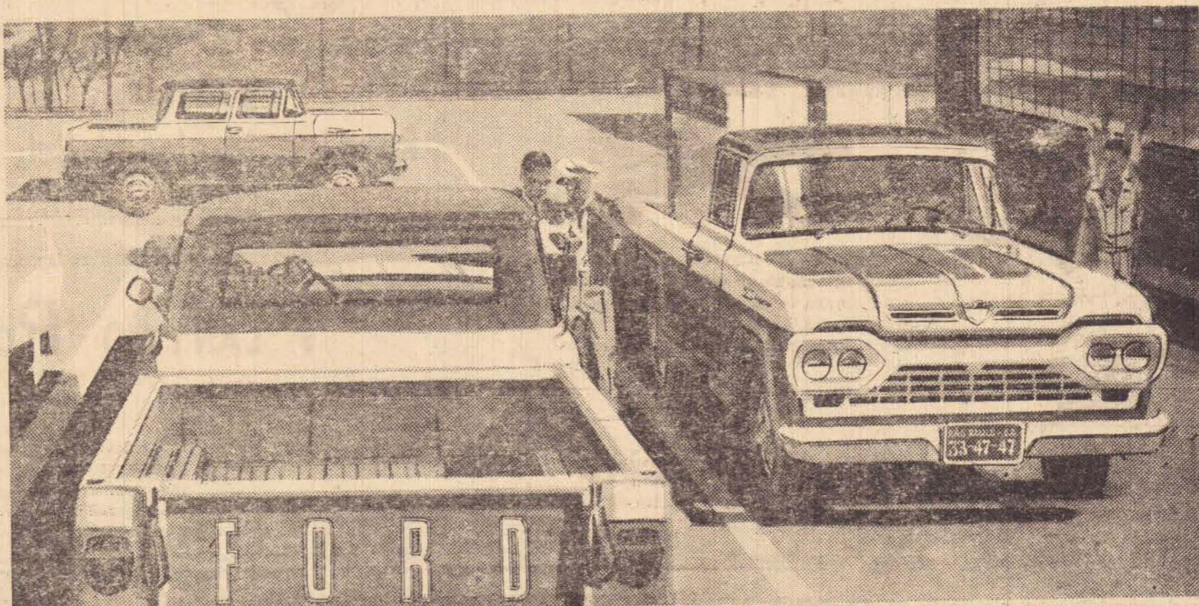
SUPER FORD F-100 — Camioneta com o conforto, estilo e desempenho dos modernos carros de passeio: cabina espaçosa, pára-brisa panorâmico, alavanca de câmbio na direção, assento e encosto de espuma de borracha. Fácil de manobrar, ágil no trânsito, ideal para entregas urbanas. Capacidade de carga: 930 kg. Motor: V-8, de 167 H.P. Distância entre eixos: 2,80 m.
