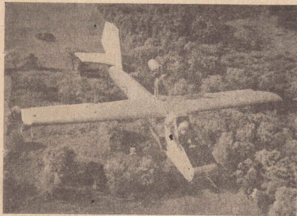
Um singular avião de estrutura inflável, desenvolvido pela Goodyear, foi proposto para uso como autômato militar sofisticado, como veículo dirigido por controle remoto ou como veículo de resgate e fuga.
