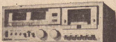
TAPE DECK CD 3700. Frontal com sistema Dolby e ajuste para Metal Tape
