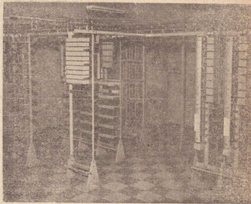
Vista interna da Central automática de Presidente Bernardes
