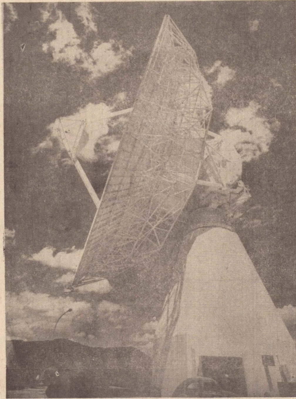
Já está funcionando a estação terrestre de satélites, construída pelo Ministério das Comunicações, em Itaboraí, sua gigantesca antena parabólica, de 30 metros de diâmetro (foto), pode ser apontada para qualquer satélite dentro de seu campo de visada, e transmitir ou receber telex, telefonia, telegrafia, e programas de TV.
