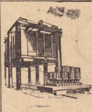
FÔRNO ELÉTRICO DE DE MALLEABILIZAÇÃO Representa a forma mais controlada de malleabilizar o ferro.
