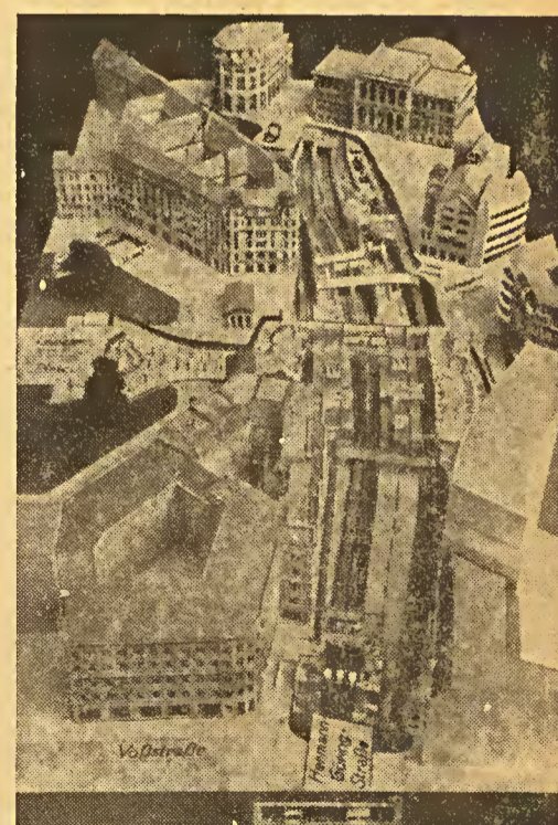
Vom Bau der Berliner Nord-Süd-S-Bahn. — Unser Bild zeigt den Modellbau des Untergrundbahnhofes Potsdamer Platz.
