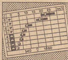
Transmissão de 8 velocidades à frente.
