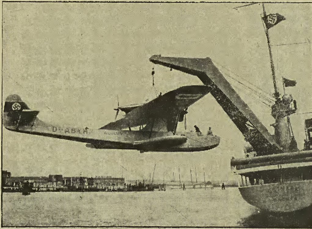
Der neue Flugzeugstützpunkt „Ostmark“. — Der am 15. April in Kiel vom Stapel gelaufene dritte deutsche Flugstützpunkt, die „Ostmark“, konnte jetzt auf seiner ersten Probefahrt seine neuen hervorragenden Eigenschaften unter Beweis stellen. Im Gegensatz zu seinen beiden Vorgängern, die im Südatlantik Dienst tun, und die umgekehrte Schiffe sind, handelt es sich hier um einen Spezial-Neubau. Auf unserem Bild sieht man die Anbordnahme eines Flugbootes.
