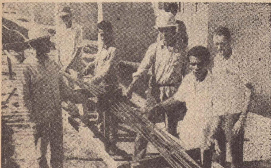
Nesta fotografia de "O Imparcial", batida por João Hirai é observado o sistema de montagem de um dos 17 cabos-tirantes que formam a sustentação da cobertura. Vemos no primeiro plano o sr. Francisco Pereira, chefe do setor técnico das oficinas da S.E.P.E. — Serviço de Engenharia e Projeto de São Paulo. Acompanha-o, nos detalhes da execução do serviço, o senhor José Menossi, mestre-de-obras do N.T.C., integrante da laboriosa equipe de "Marinho & Nishimura".
