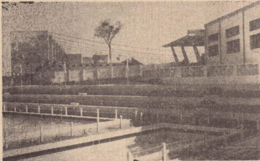
Aqui está uma visão das obras do "colosso da Washington Luiz", já com os cabos-tirantes instalados. Cada um deles pesa exatamente 300 quilos. E o conjunto sustentará as 420 telhas em "fiberglass" que cobrirão a sede-social.
