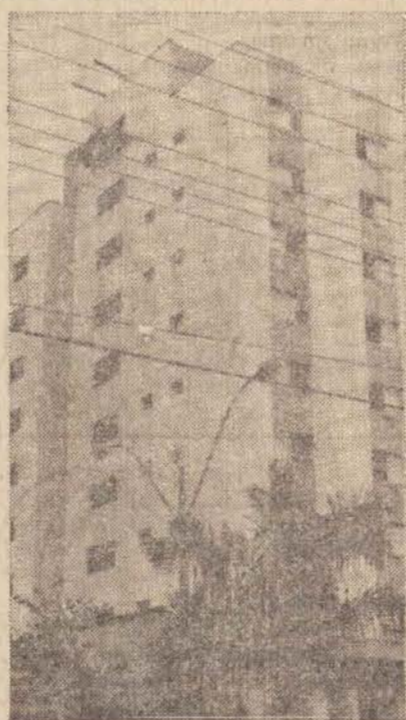
Edifício "Sergio Lopes da Silva" Av. Washington Luiz, 142 10 pavimentos 16 apartamentos 16 boxes-garagem área construída: 3.610,20 metros quadrados (empreendimento em obras) unidades à venda previsão de entrega: 1980
