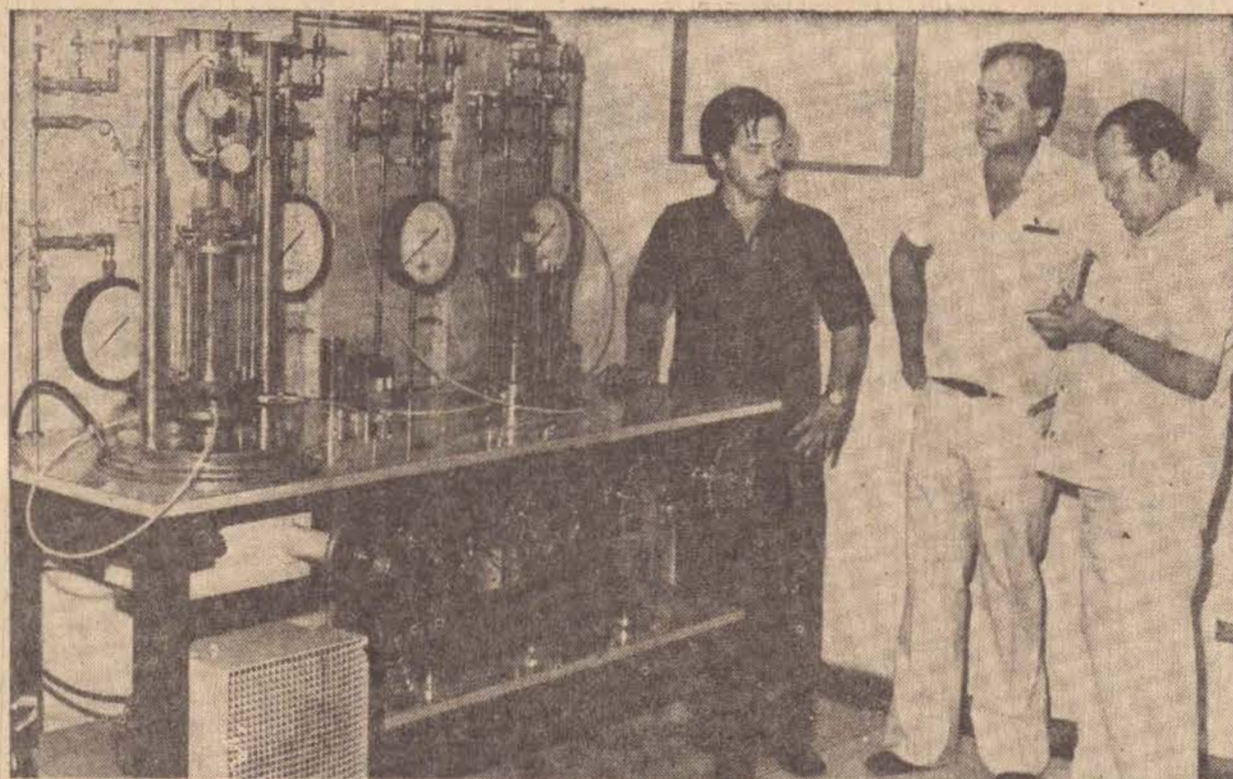
Ao lado do prof. Agripino de Oliveira Lima Filho, técnico da Faculdade de Engenharia Civil, dr. João de Ensaio Triaxial, um dos dez existentes em todos de orientação e ensino a reportagem ouviu os esclarecimentos do diretor. Carlos Rela, acerca do funcionamento do Conjunto o Brasil e tido como um dos principais equipamentos acerca da mecânica do solo.
