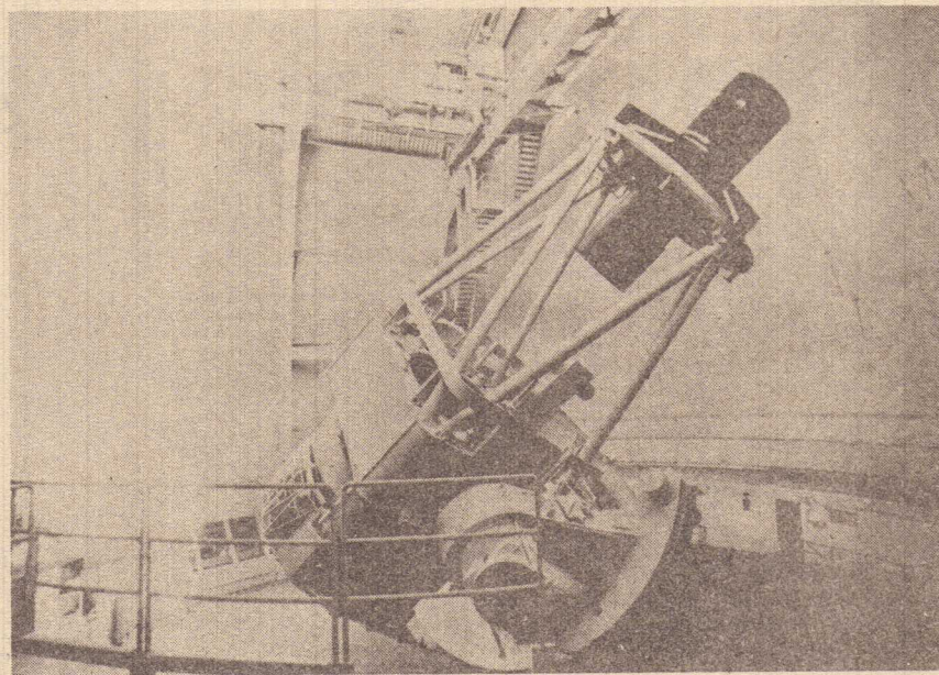
▲ Um telescópio moderno como este, se lançado ao espaço, poderá ampliar as fronteiras do homem.
