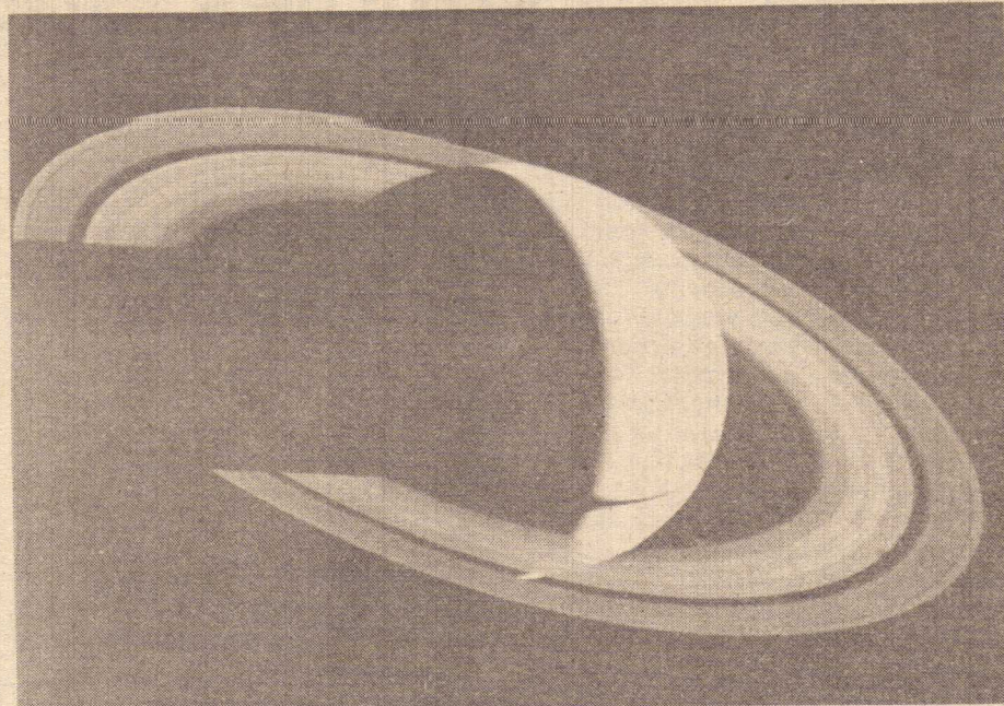
▲ Saturno e seus anéis, um dos planetas já pesquisados pelo homem.
