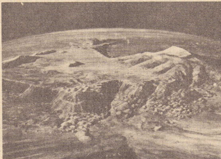
▲ A superfície de Vênus, segundo a concepção dos cientistas.
