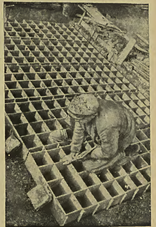
Deutsches Pflaster erobert die Welt. — Nicht nur in deutschen Städten, sondern auch im Auslande gehen wir auf „deutschem Boden“. Durch ein einzigartiges Verfahren wird bei der Verschmelzung des Mansfelder Kupferschiefers abfallende Kupferhochfeuschlacke zu Pflastersteinen verarbeitet, die dann in die Welt exportiert werden. Die Gießgrube zur Herstellung des Mansfelder Pflastersteines wird mit der Hand hergestellt.
