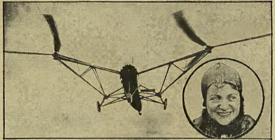
Hubschrauberrekord von Flugkapitän Hanna Reitsch. — Eine neue Höchstleistung für Hubschrauber im Streckenflug ohne Zwischenlandung wurde von Flugkapitän Hanna Reitsch zwischen Stendal und Berlin-Tempelhof mit 108 Kilometer aufgestellt. — Das Rekordflugzeug ist der Hubschrauber von Prof. Focke „SW 61“, mit dem kürzlich eine Reihe anderer Höchstleistungen erzielt worden sind, darunter ein Streckenflug von 16 Kilometer, der jetzt von Flugkapitän Hanna Reitsch auf 108 Kilometer ausgedehnt werden konnte.
