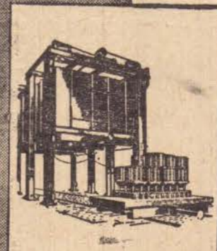
FORNO ELÉTRICO DE MALEABILIZAÇÃO
