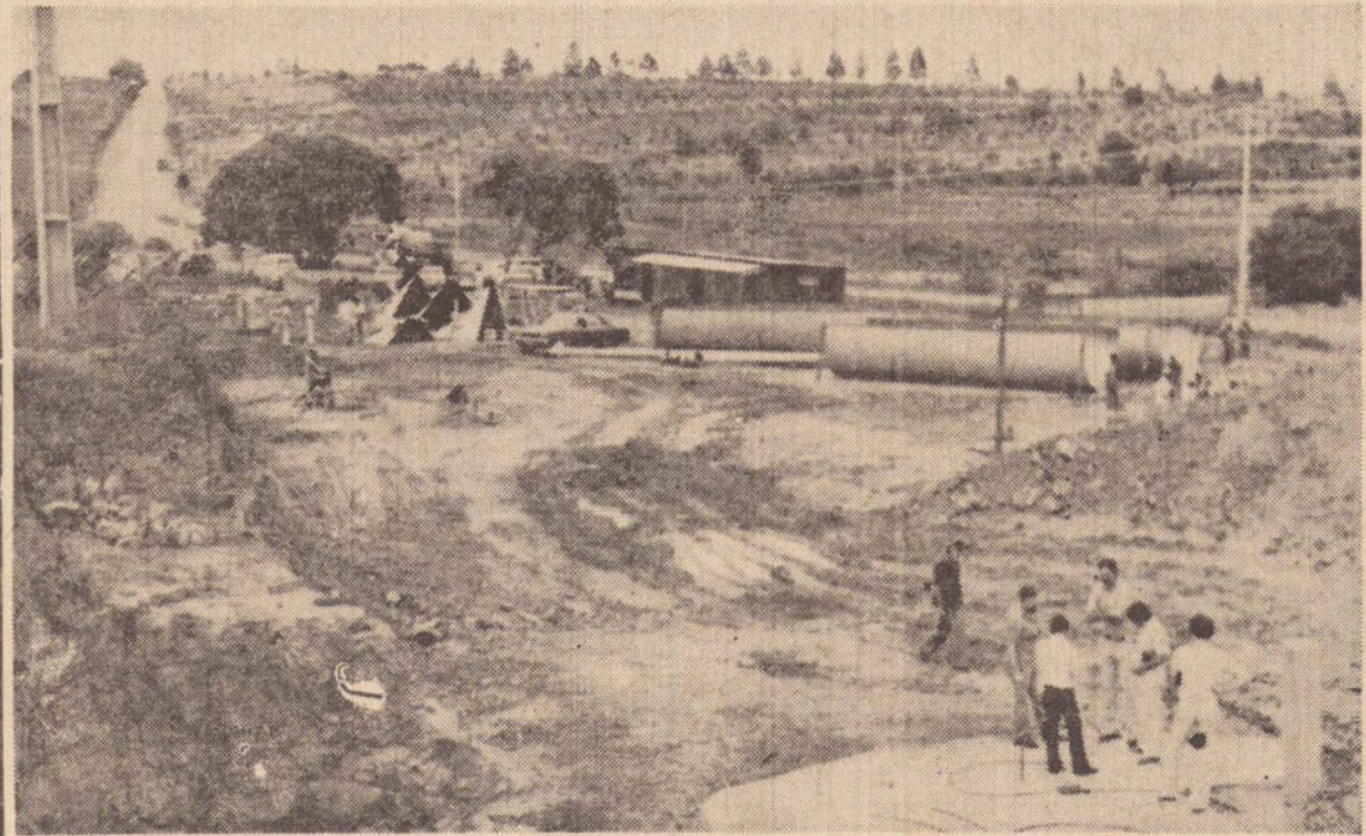
Vista parcial da área onde está sendo construída a grande usina da Concrebrás S.A. — Engenharia de Concreto.
