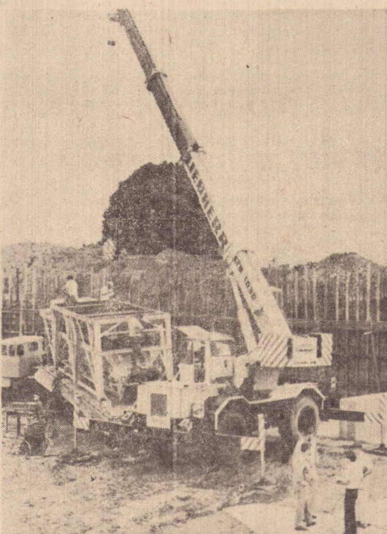
Momento em que o guincho desce a pesada máquina da usina Concrebrás, sob as vistas dos diretores, funcionários e da reportagem. Fotos de Luiz Sant'Clair.
