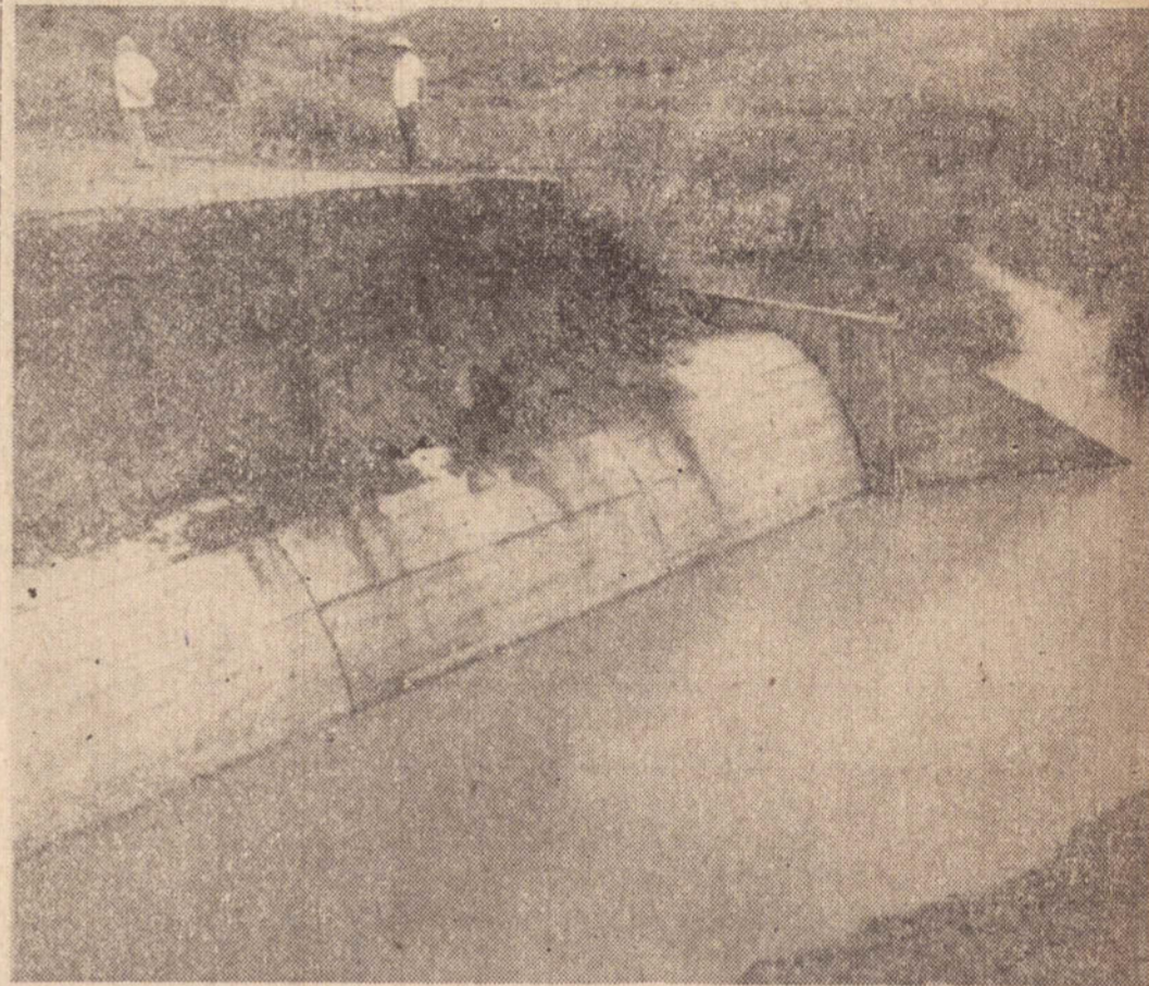
A imensa galeria sob o asfalto no km. 586 não conseguiu dar vazão ao gigantesco volume d'água acumulado durante apenas 3 horas de chuvas naquela área do município de Presidente Bernardes.
