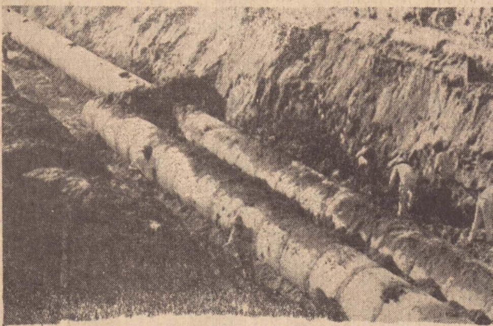
Construção da rede de galerias na bacia Vila Senhor Bonfim
