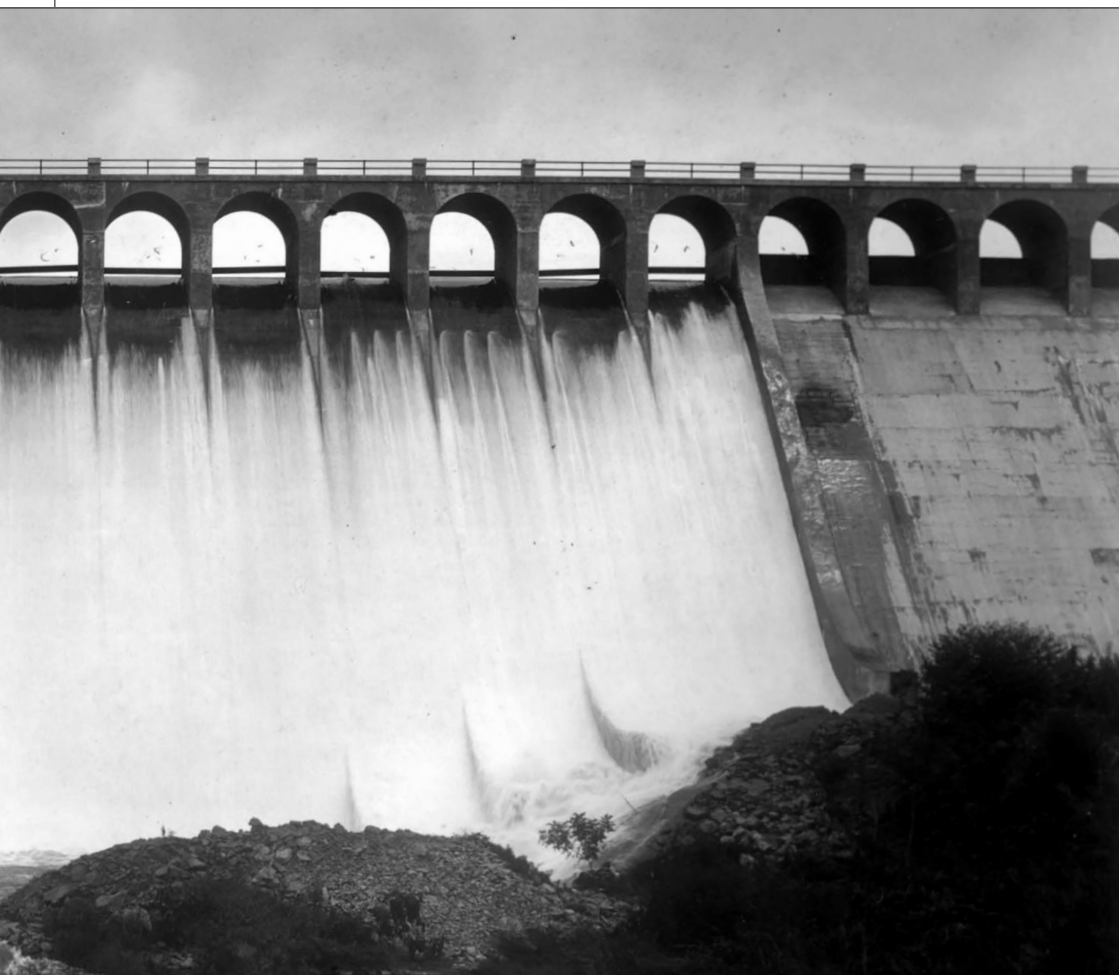
(ao lado) Usina Hidrelétrica Itupararanga. Votorantim – SP. Fevereiro, 1917 (Foto: Guilherme Gaensly)
