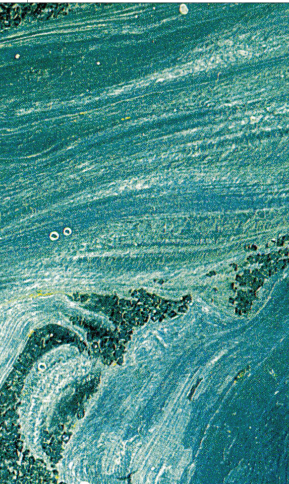
Picnodontídeo (Ostreida). Bacia de Sergipe-Alagoas, Albino, Formação Riachuelo, Carapeba
