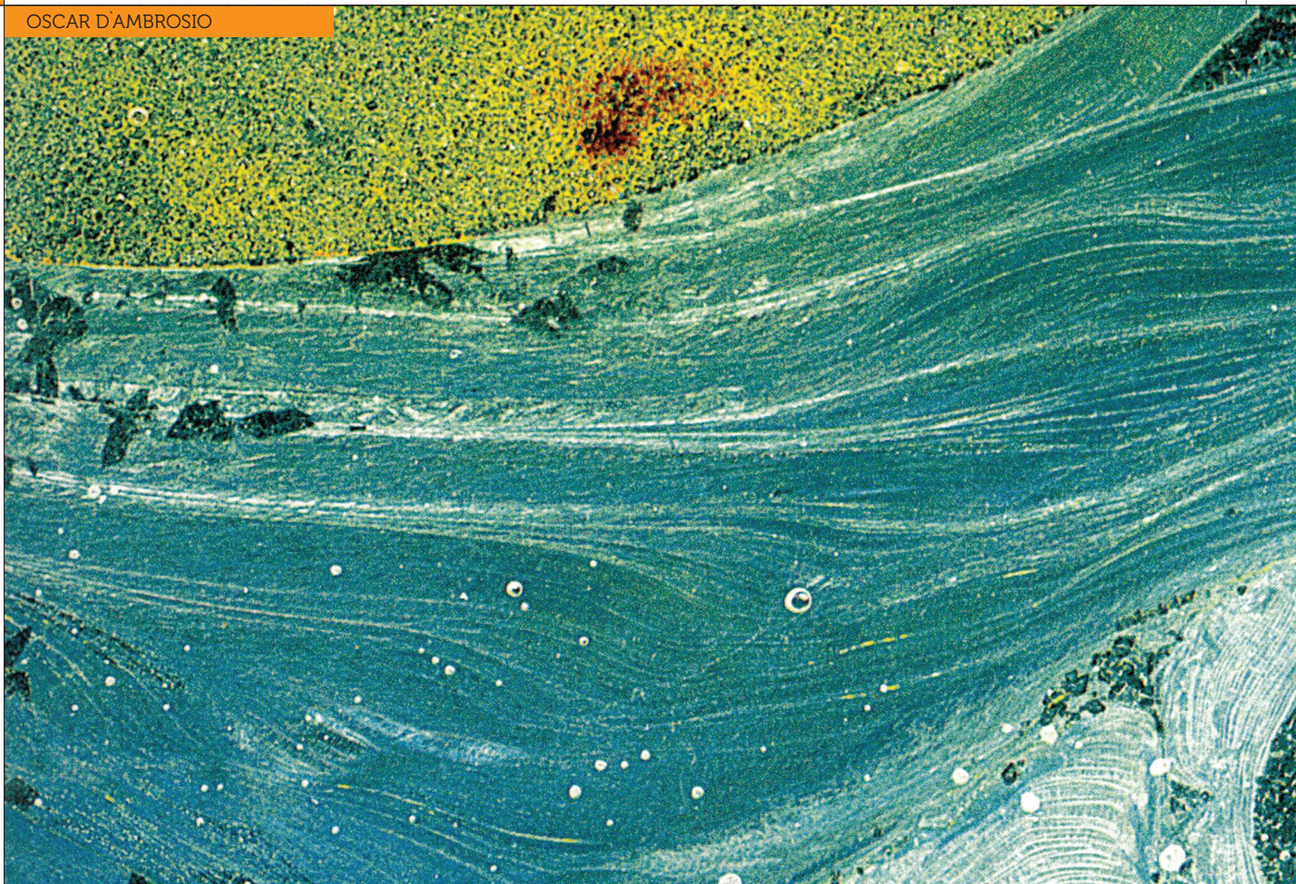
Grainstone oolítico. Destaque para Neomeris em núcleo de oolide, ambiente tropical, agitado. Bacia de Sergipe-Alagoas, Albino, formação Riachuelo, Usina Pinheiro
