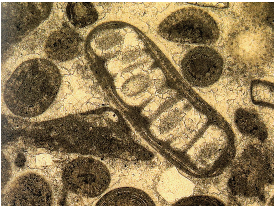
Grainstone oolítico. Destaque para Neomeris em núcleo de oolide, ambiente tropical, agitado. Bacia de Sergipe-Alagoas, Albino, formação Riachuelo, Usina Pinheiro
