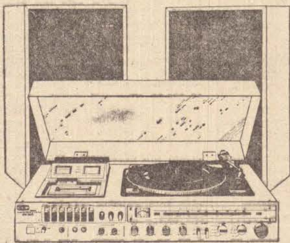
SHC-5300 Centro Musical Estereofônico. Conjunto tipo 3 em 1, com sintetizador de 4 faixas AM, FM, Estéreo/Mono, OC1 e OC2; Medidor de sinal; Muting; Toca-discos Belt Drive com retorno automático; Cassete com Dolby NR; Seleção de fitas (Normal e CrO2); Auto Stop; VU's de níveis; Potência de saída: 80 watts. Acompanham caixas acústicas CL-55.
