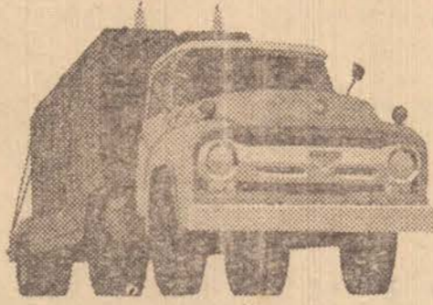
FORD F-600, Diesel, de 128 H.P. — chassis de 148", cavalos-mecânicos para 12 t.
