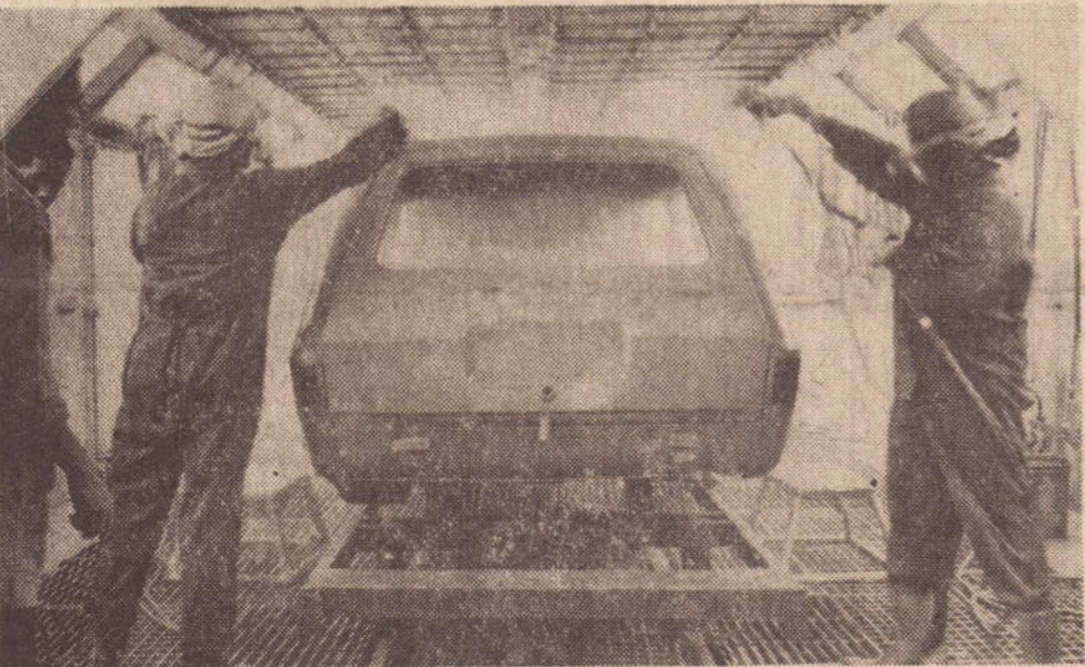
Depois de fosfatizada, a carroceria entra no tunel de pintura e na estufa.
