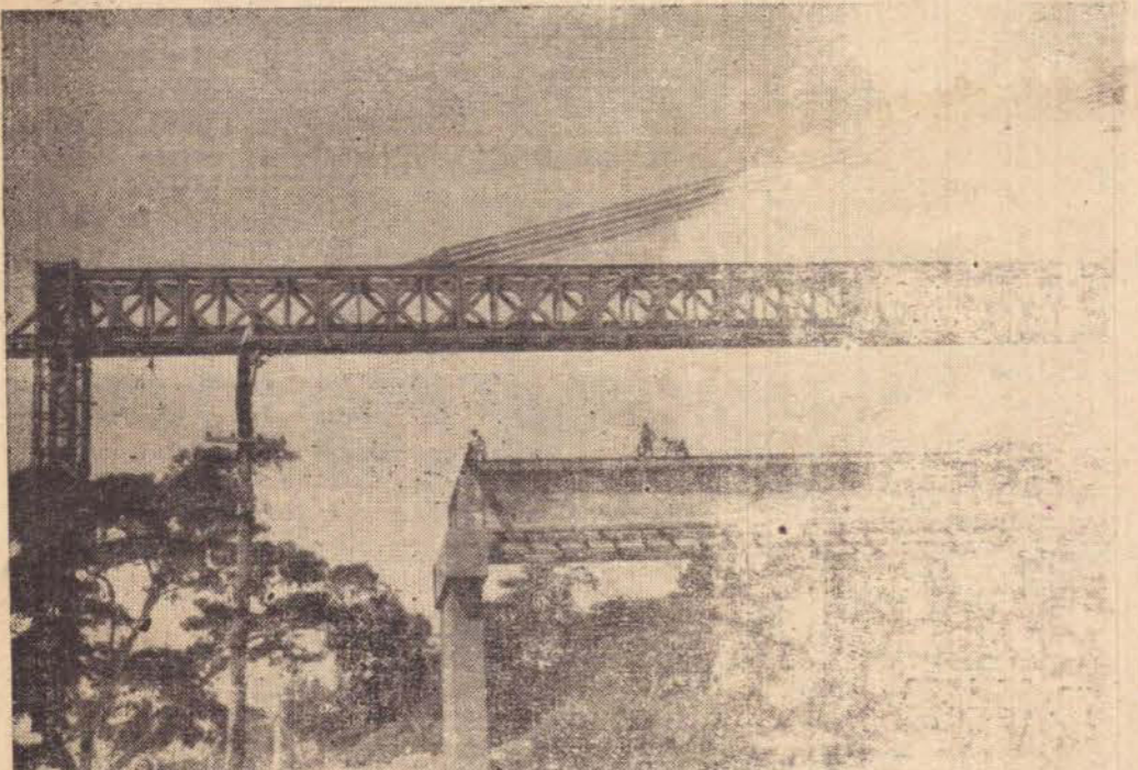
Na foto acima os leitores podem observar as gigantescas obras da Ponte Interestadual sobre o Rio Paraná, cujos dados de atualidade podem ser analisados na reportagem de Altino Corrêa sobre o último pilar construído.
