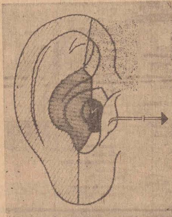
Na parte escura do desenho, está a área sensível que produz estímulos de nervos craniais.
