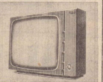
Modelo B-140, Preto e Branco, 61 cm (24 polegadas). Totalmente transistorizado. Controles lineares deslizantes. Móvel em madeira de lei. Funciona em 110, 127 e 220 volts. Imagem inabalável, garantida pelo DS-388.
