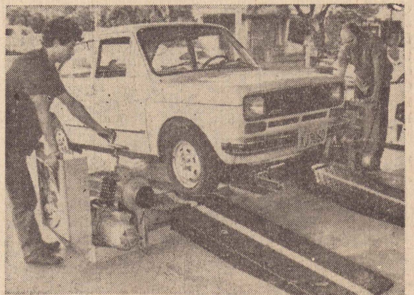
O "Shock Tester" é uma exclusividade dos Escapamentos Ipiranga.
