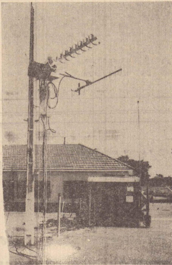
Uma antena do sistema de telemetria, indica a posição do balão no espaço.
