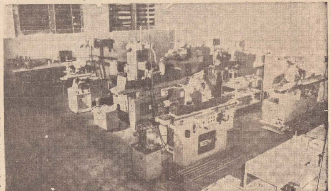
A seção de retífica, num outro aspecto parcial tomado no interior da PRUDENTRATOR. Ressalte-se que a maioria das máquinas que formam este complexo são importadas.
