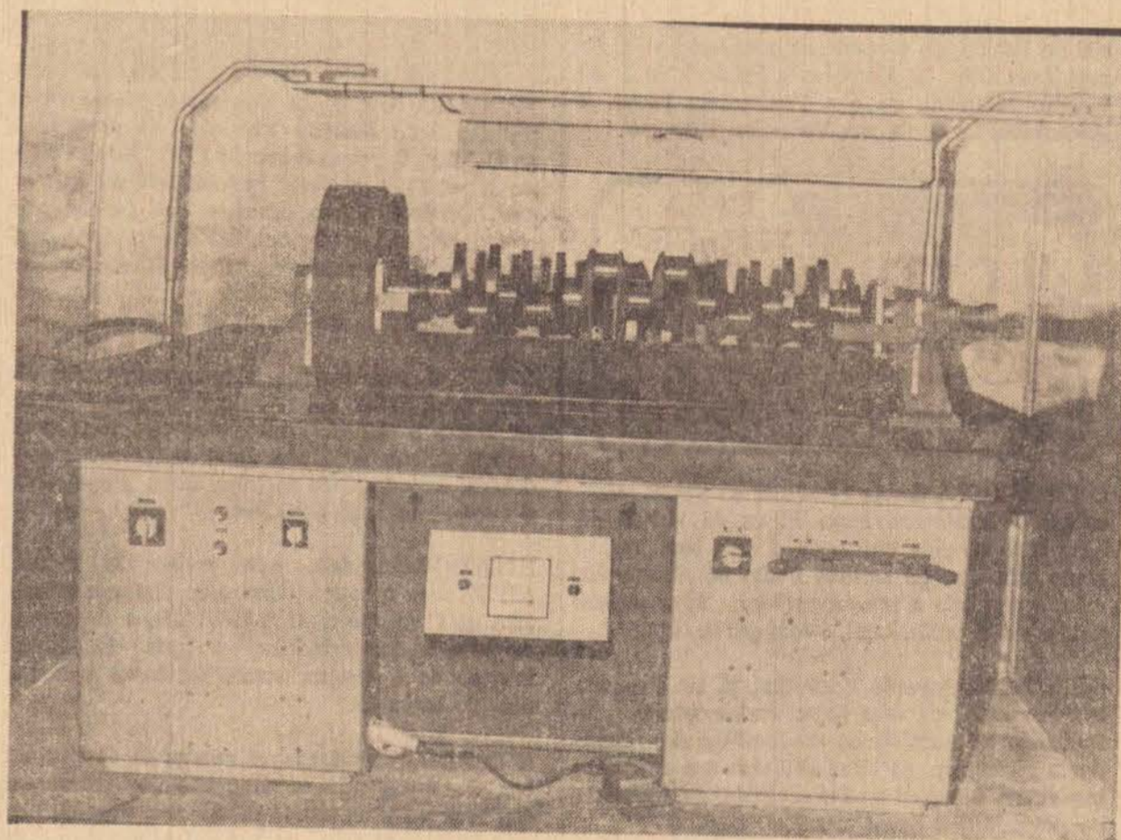
Esta é a máquina detetora de trincas, em operações na Retimar-Motores, a Av. Brasil, 2.975.
