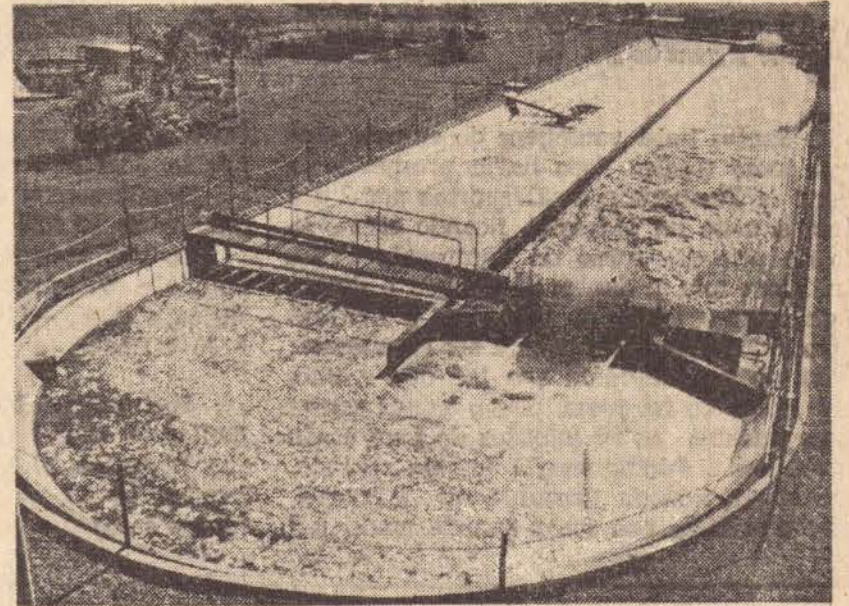
Neste tanque inicia-se o tratamento de efluentes com a injeção de ar na água.
