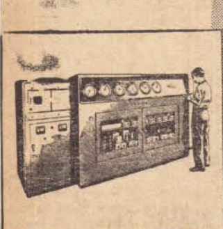
ESPECTRÔMETRO Permite a análise de ferro fundido antes do vasamento.
