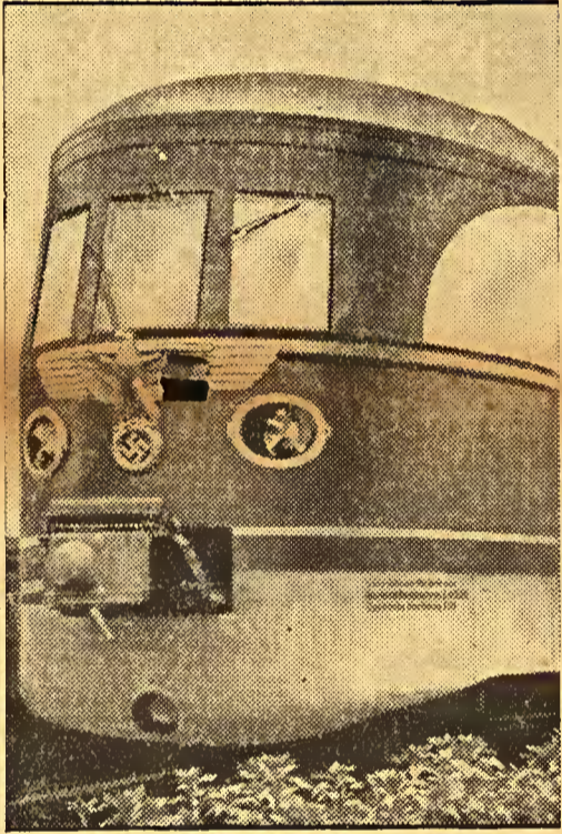
Ein neuer „Fliegender“. — Ein neuer Triebwagen der Deutschen Reichsbahn, der auf der Strecke Berlin-Köln in Dienst gestellt wird. Der Wagen, der mit 2 Diesel-Elektromotoren zu je 600 PS ausgestattet ist, erreicht eine Geschwindigkeit von 160 Kilometer in der Stunde. An der Front trägt er das deutsche Hoheitszeichen.
