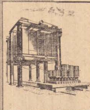
FORNO ELÉTRICO DE MALEABILIZAÇÃO Representa a forma mais controlada de maleabilizar o ferro.
