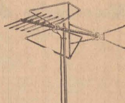
ANTENA PARA TV Super reforçada, apresenta melhor ganho nos canais baixos.
