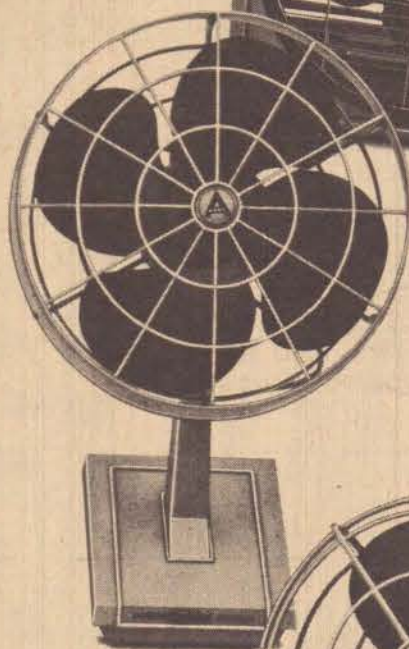
Ventilador Arno Para qualquer ambiente. Diâmetro 30 cm, com três velocidades, oscilante. Hélice azul e arco plástico para maior concentração do ar.
