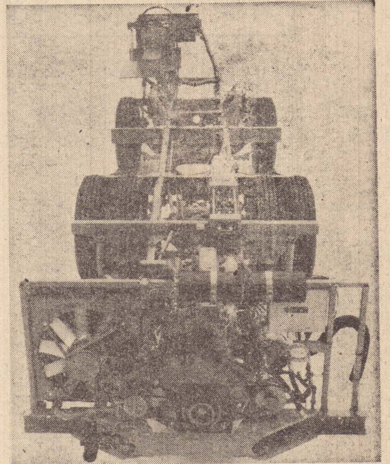
Chassi do ônibus K 112, pronto para receber a carroçaria.
