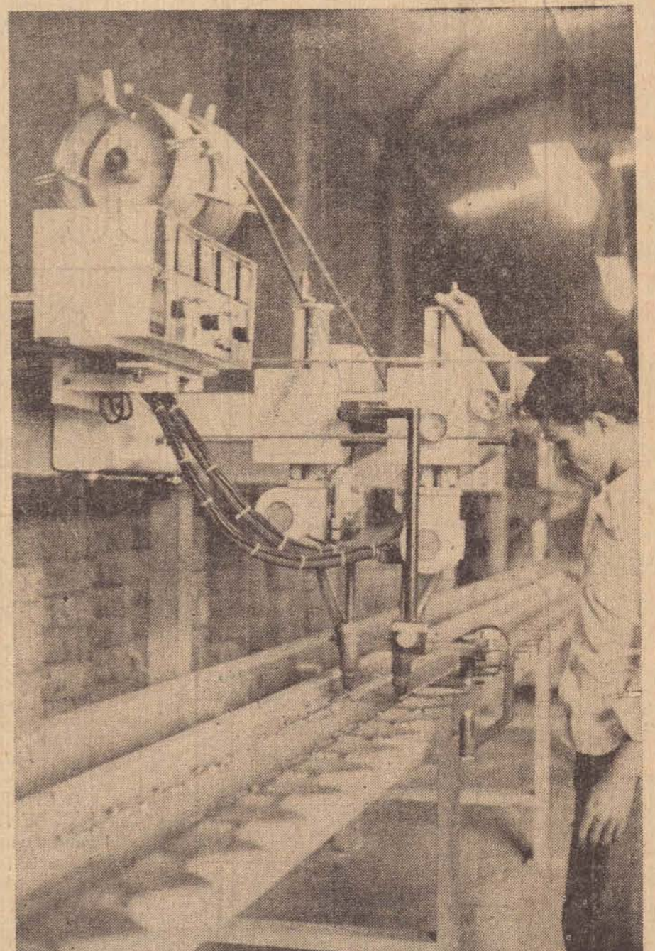
Esta possante máquina, de fabricação nacional, cuida, sob processo eletrônico, da restauração das peças através a soldagem. Apenas um operário mobiliza o equipamento, constituindo-se a máquina numa das importantes peças do complexo de TRATORTECNICA.
