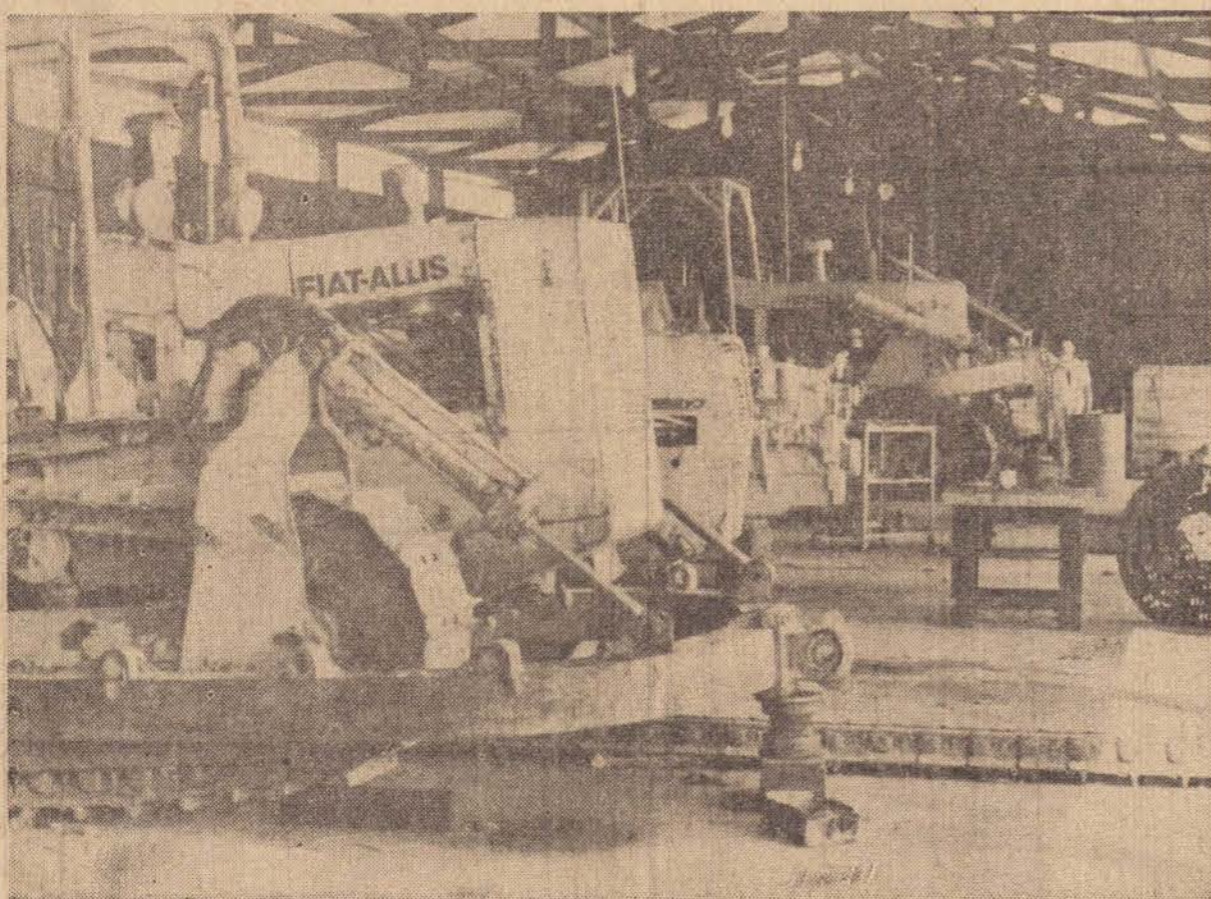
Em amplo galpão, com divisões numeradas, a TRATORTECNICA realiza, com notoriedade, os serviços de restauração de tratores de esteiras, operando preferencialmente com os da linha Fiat Allis, conforme se pode ver nesta fotografia que mostra, parcialmente, a oficina de montagem e desmontagem.
